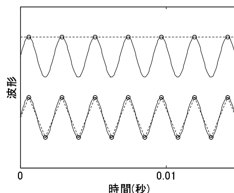
図3 サンプリング定理の説明。サンプリング間隔が波長の1/2で、かろうじて波形の変化に追従できる。
